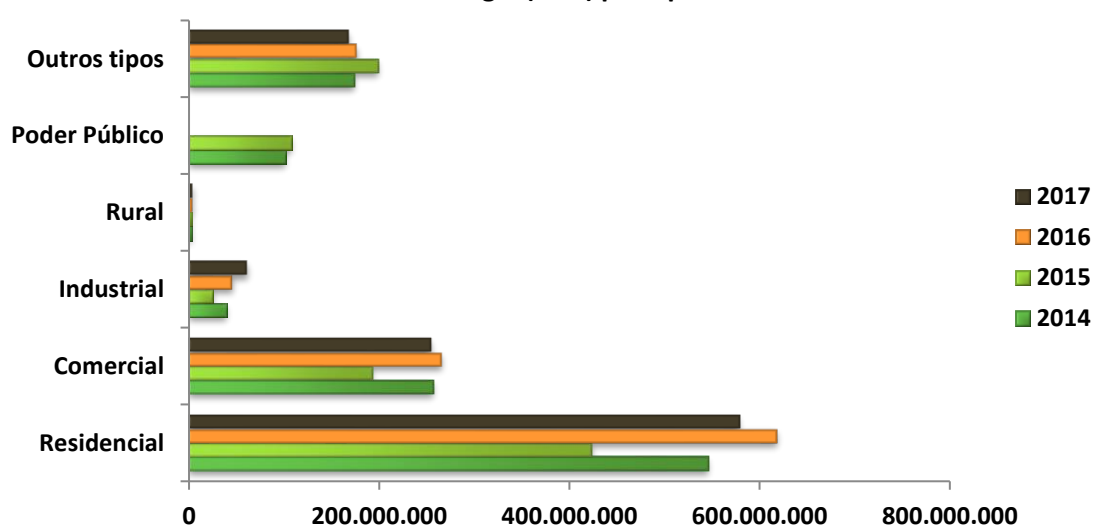
Gráfico 7.1 - Consumo de energia (kwh) por tipo de usuário - 2014 - 2017
